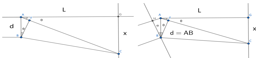
(a) 夫琅禾费衍射光路图：入射光垂直于光栅 AB；衍射光大角度斜射光屏。 (b) 改进的衍射光路图：入射光斜射光栅；衍射光小角度斜射光屏。
