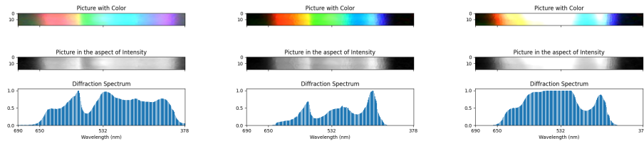
(a) 日光: 波段较宽而且连续
